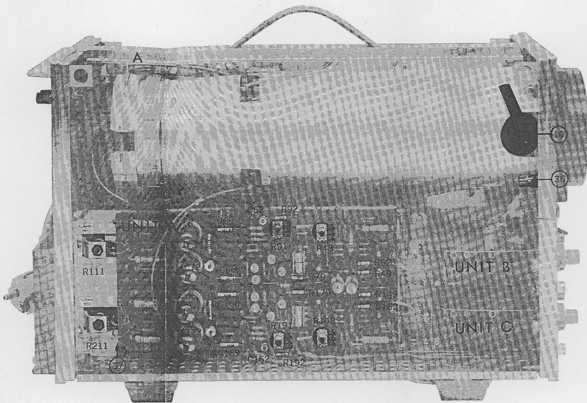
Fig. 6. Rechter-zijaanzicht
