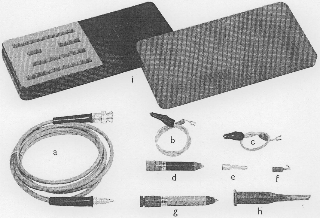
Fig. 17. Meetkopset
