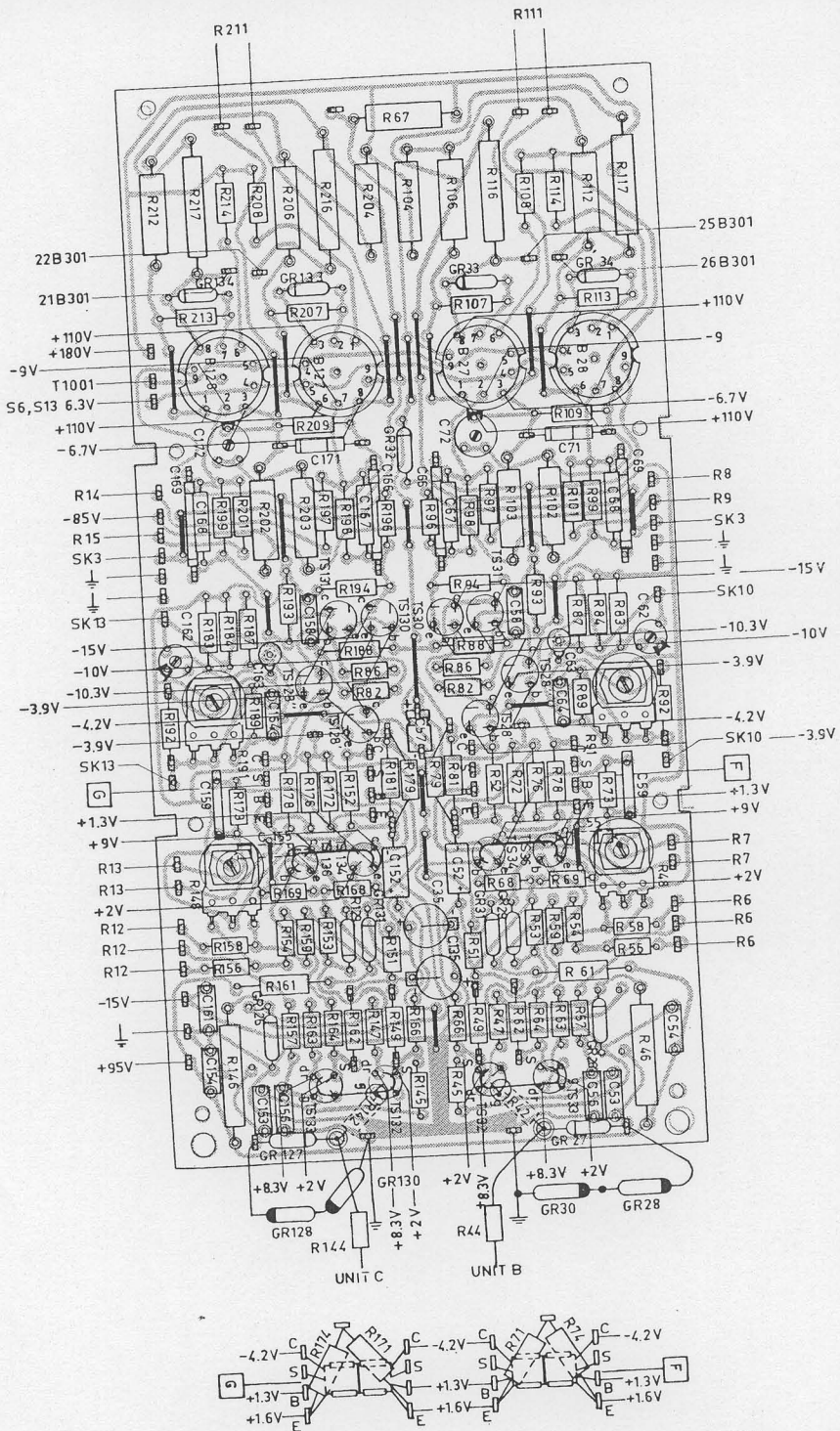
Fig. 26. Gedrukte-bedradingsplaat A
