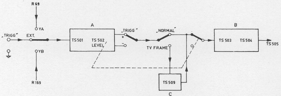
Fig. 8. Blokschema - Triggerimpulsvormer
