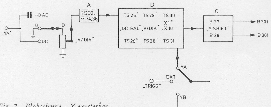
Fig. 7. Blokschema - Y-versterker
