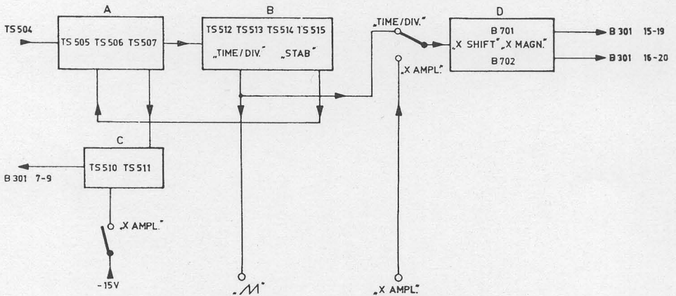
Fig. 9. Blokschema - Tijdbasisgenerator en X-versterker
